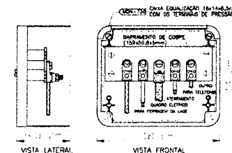
2 DETALHE DO ATERRAMENTO DO SPDA SEM ESCALA
