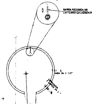
RESERVATÓRIO 33m 3 CISTERNA 4,5m 3 CORTE NÍVEL 3
