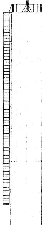
RESERVATÓRIO ELEVADO 12 m 3 CISTERNA 4,5 m 3 VISTA LATERAL 2
