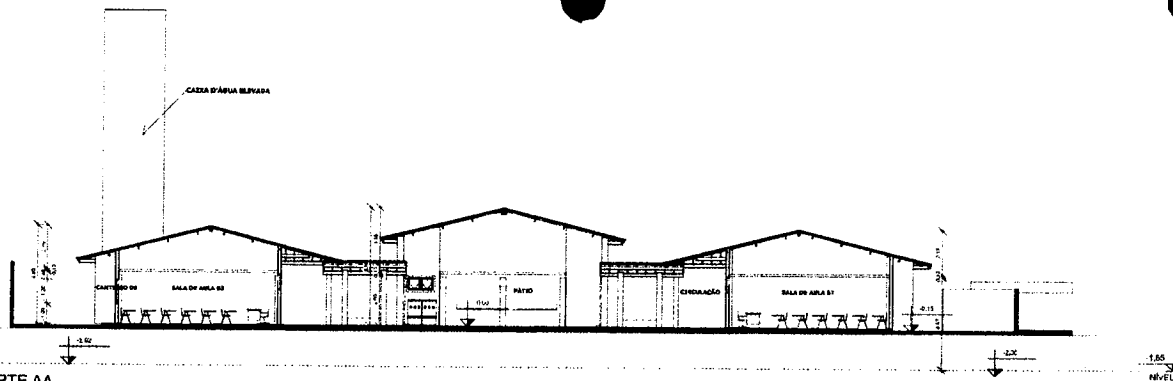
1 CORTE AA 1:125
