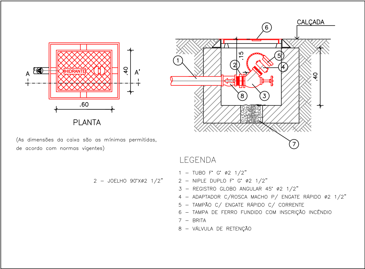
Detalhe hidrante de recalque Sem escala
