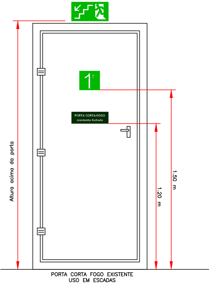
Detalhe iluminação de emergência Sem escala
