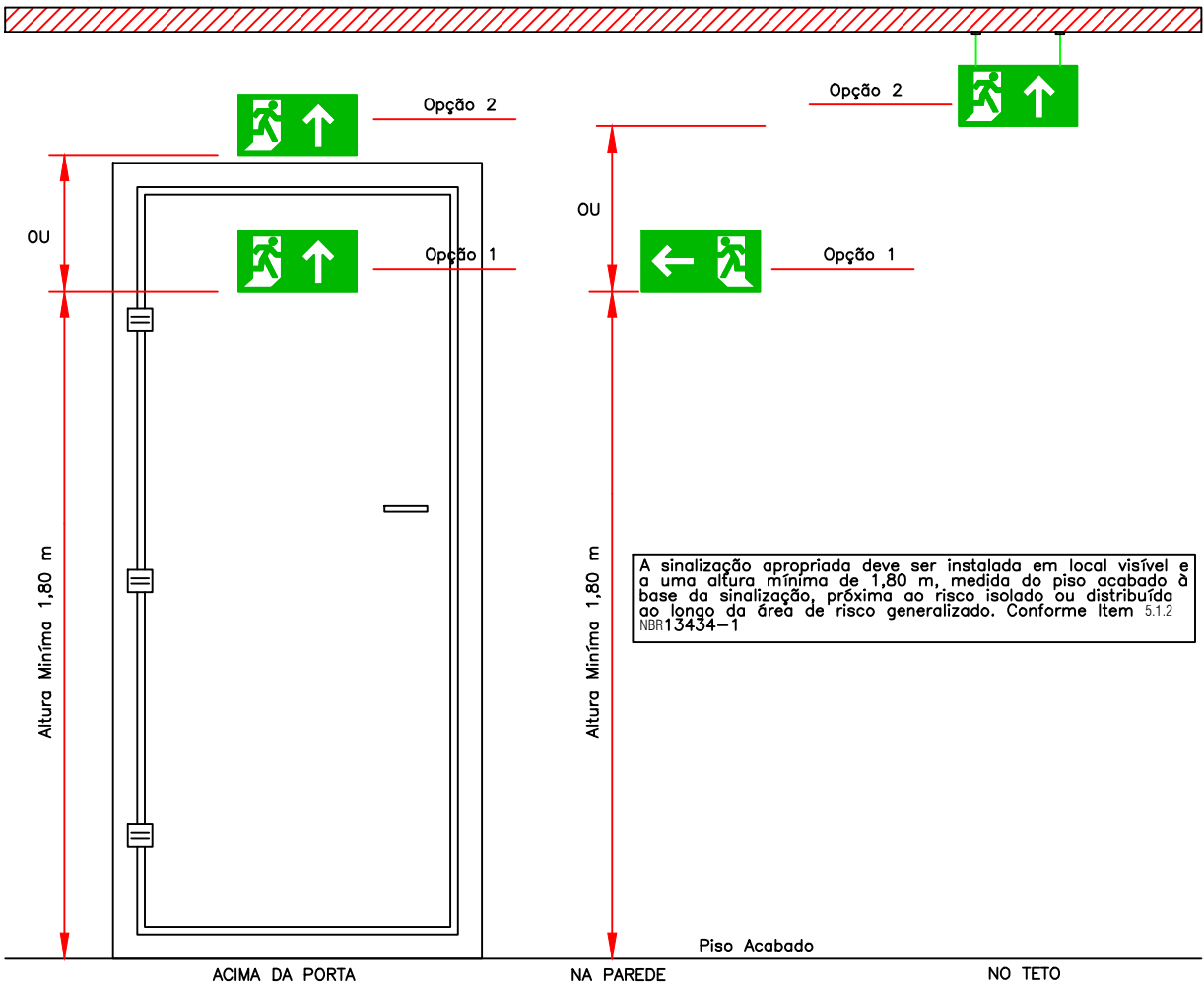
Detalhe sinalização de emergência Sem escala
