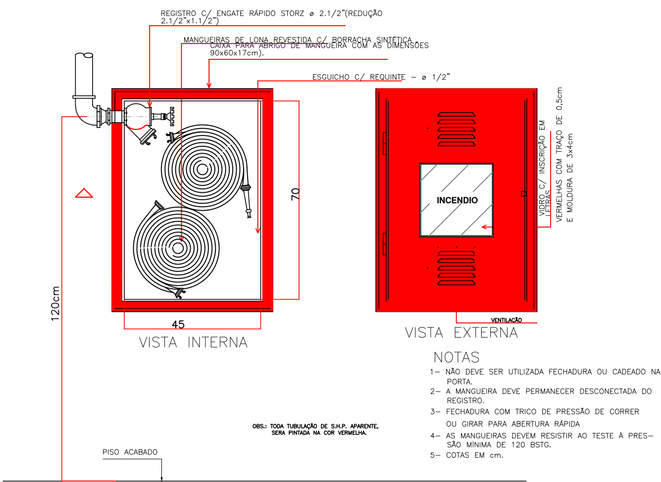
Detalhe hidrante simples Sem escala
