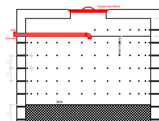
SUMIDOURO CORTE - ESC. 1:25
