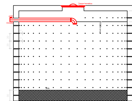
SUMIDOURO CORTE - ESC. 1:25
