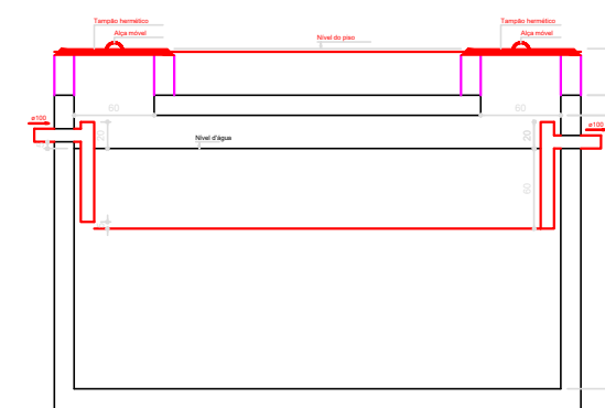
TANQUE SÉPTICO CORTE - ESC. 1:25
