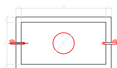
TANQUE SÉPTICO PLANTA BAIXA - ESC. 1:25
