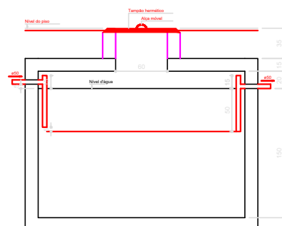
TANQUE SÉPTICO CORTE - ESC. 1:25
