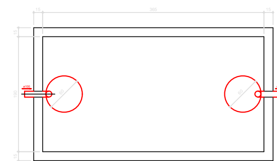
TANQUE SÉPTICO PLANTA BAIXA - ESC. 1:25
