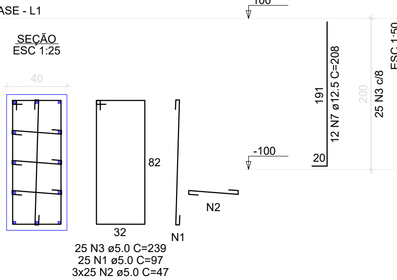
P2=P3=P4=P5=P6=P9=P10=P11=P12= =P13 BASE - L1 SEÇÃO ESC 1:25
