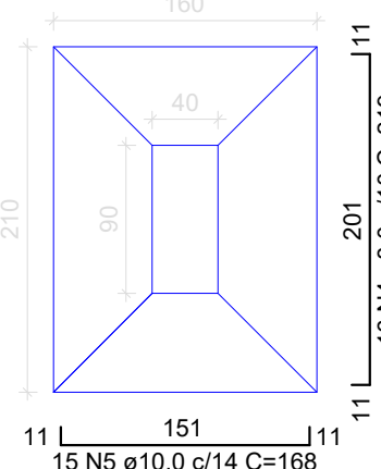
S1=S7=S8=S14 PLANTA ESC 1:50
