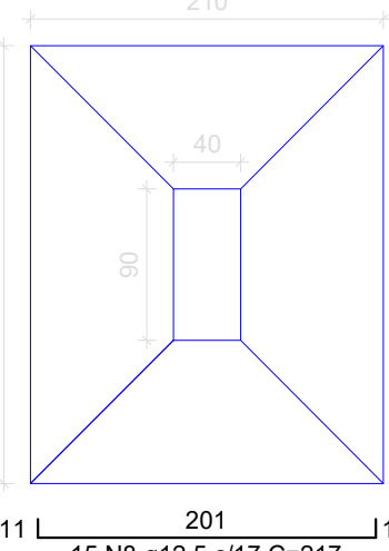
S2=S3=S4=S5=S6=S9=S10=S11=S12=S13 PLANTA ESC 1:50
