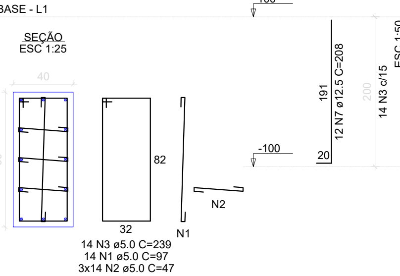
P1=P7=P8=P14 BASE - L1 SEÇÃO ESC 1:25
