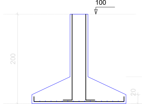
CORTE ESC 1:50
